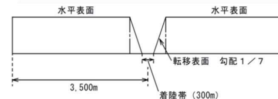
制限表面の断面図 断面B-B'
