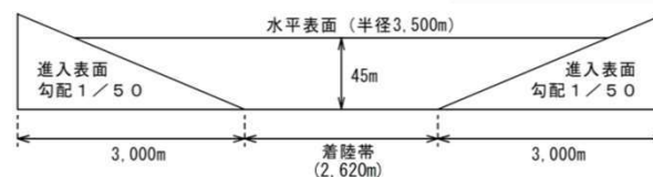
制限表面の断面図 断面A-A'
