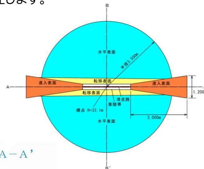
制限表面平面図
